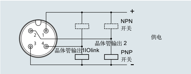
SITRANS LCS050 接线图
